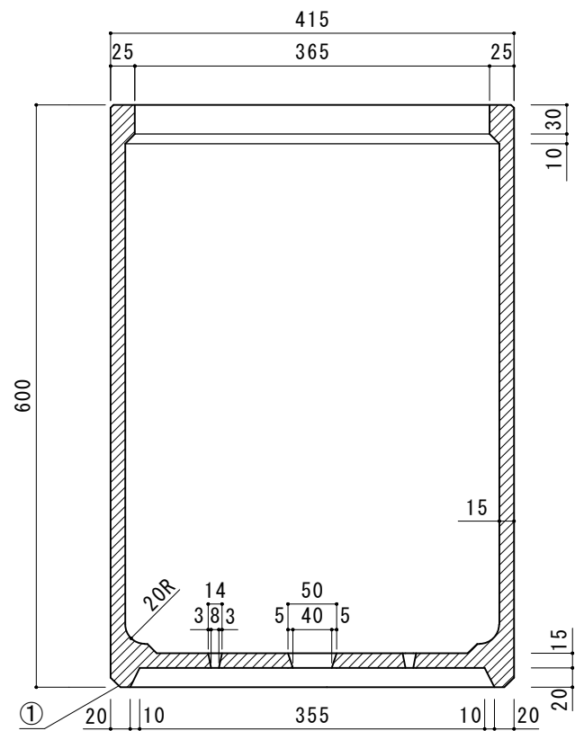
【A-A' 断面図】
