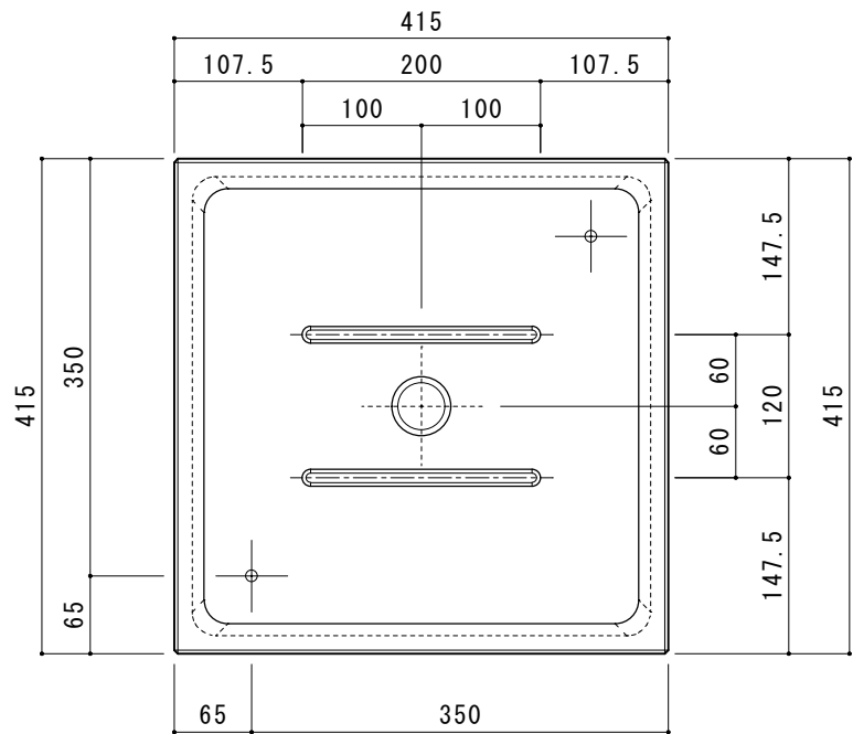
【上面図】
