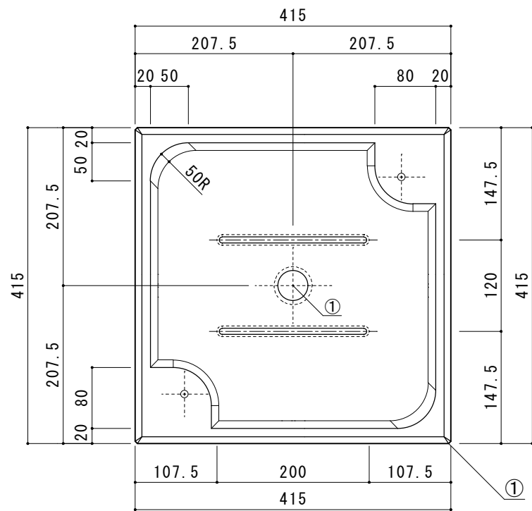
【底面図】
